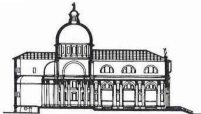
SECCIÓN A
