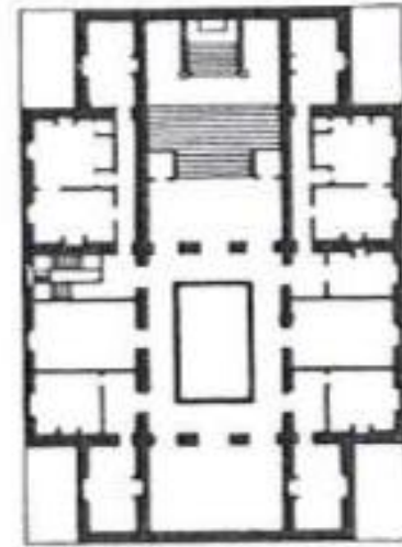
PLANTA SUPERIOR
