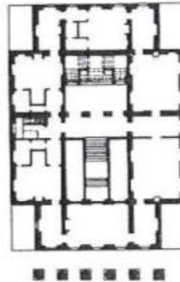
PLANTA INTERMEDIA
