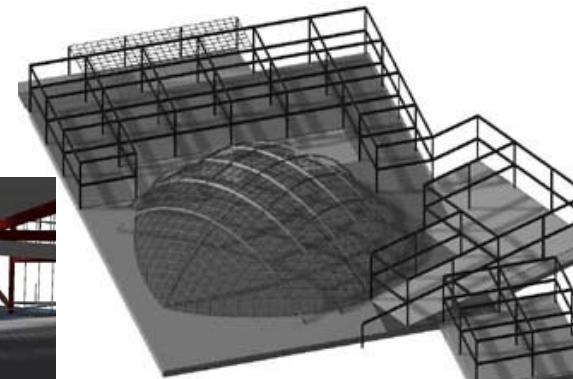
Isométrica da estrutura
