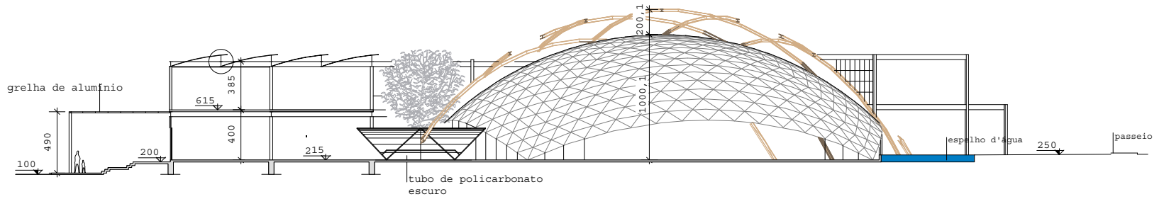
Seção longitudinal
