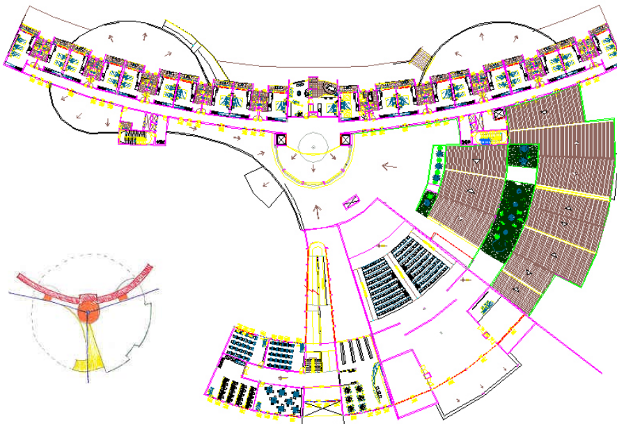
FIG 18: Planta Baixa Mobiliada Pav. Tipo, sem escala.
